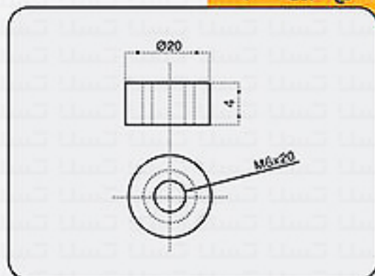
نوع قطبین (mm)
