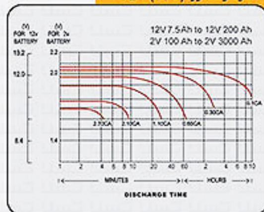
نمودار دشارژ ۲۵°C (۷۷°F)
