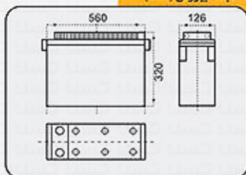
ابعاد بیرونی (mm)
