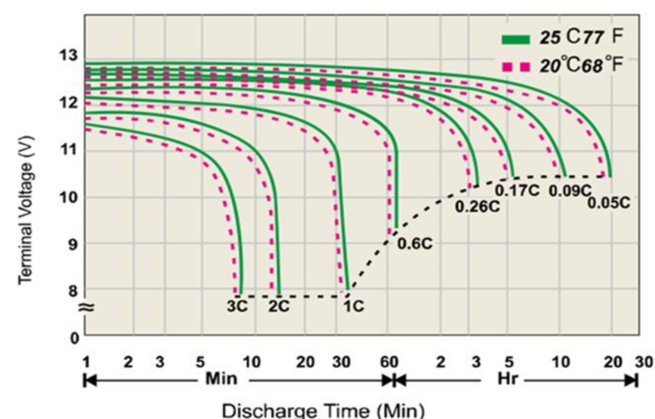
نمودار دشارژ
